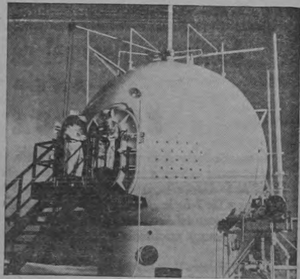
Los técnicos de la Esso remueven equipos de una esfera de 18 pies en uso para pruebas de combustibles sólidos para cohetes. La nueva esfera de pruebas fue terminada de construir recientemente en Linden, New Jersey, por la Esso Research and Engineering Company. Esta Compañía trabaja bajo contrato del gobierno americano en el desarrollo de nuevos combustibles sólidos para cohetes.
